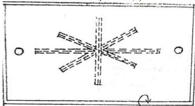
M.S. SQ. BAR 32 X 32 MM X 2 NOS
